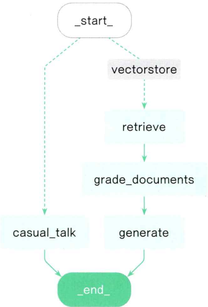
RAG가 필요한지 판단하고 동작하는 랭그래프의 구조
